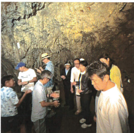
不動窟 (鍾乳洞) 見学
